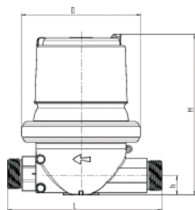
620-C DN15
