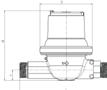
620-C DN20
